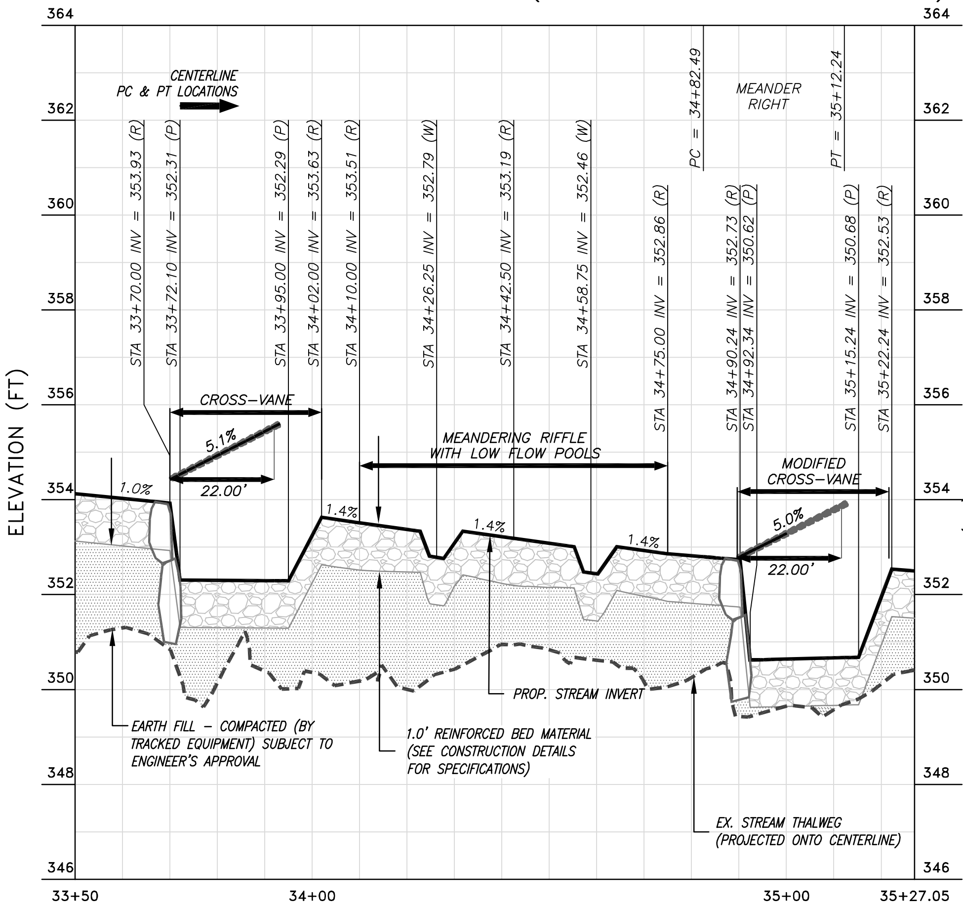
LONGITUDINAL PROFILE - REACH 4A (STA 33+50 TO STA 35+27.05)
