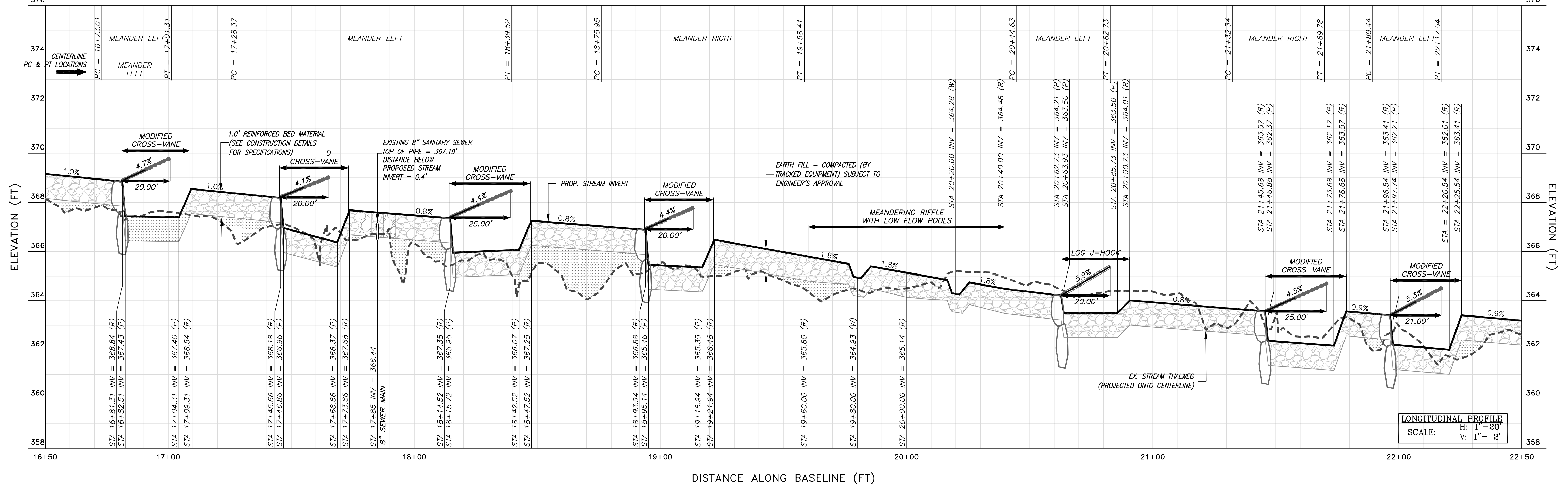
LONGITUDINAL PROFILE - REACH 4A (STA 16+50 TO STA 22+50)
